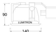
LMDL-8A Cut-out 120mm.
